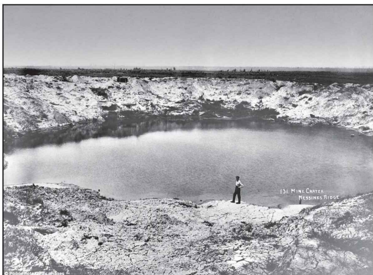
Salah satu kawah dari 19 kawah bekas ledakan dari Pertempuran Messines 1917. (sumber gambar: www.ww1.co.uk )
