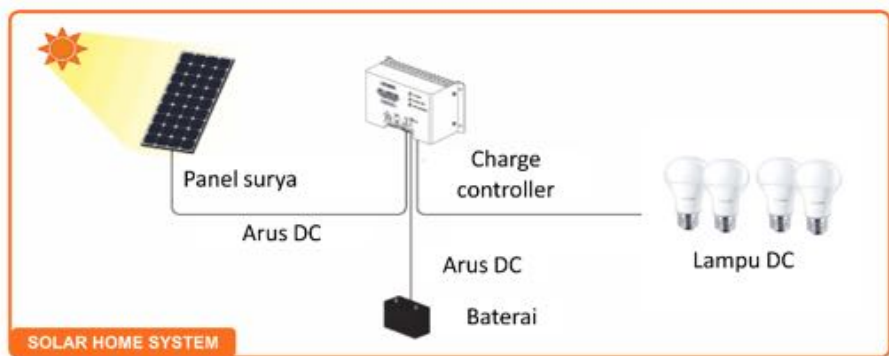
Gambar 7 Contoh Aplikasi Pembangkit Listrik Tenaga Surya
