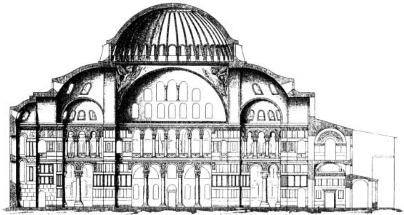
St. Sophia tampak dari samping
