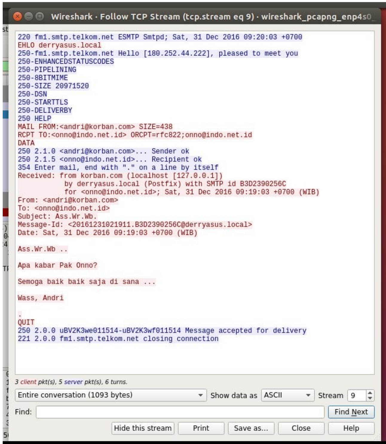
Gambar 6: Hasil penyadapan komunikasi e-mail
